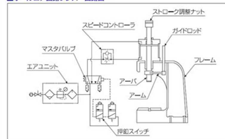
■オールエア回路プレス 回路図
